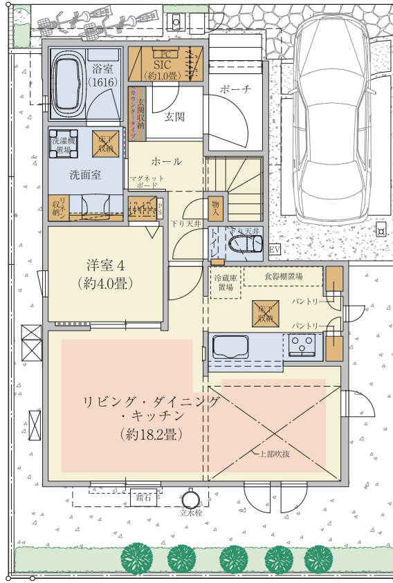
【1階平面図】
