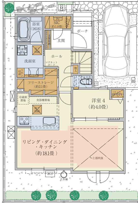
【1階平面図】
