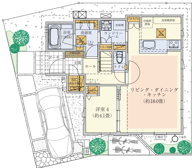
【1階平面図】
