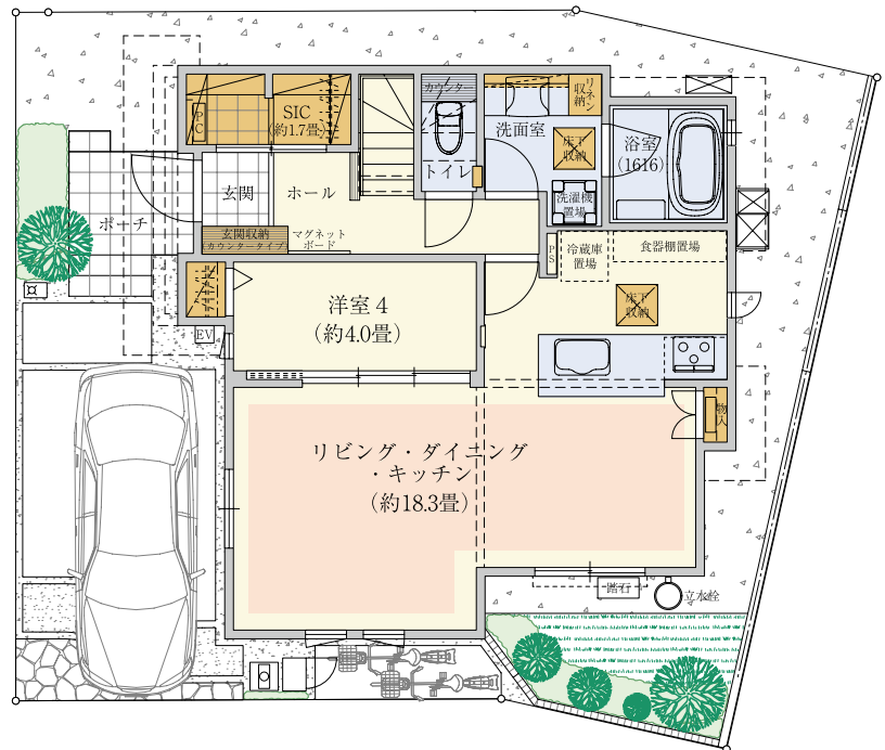
【1階平面図】
