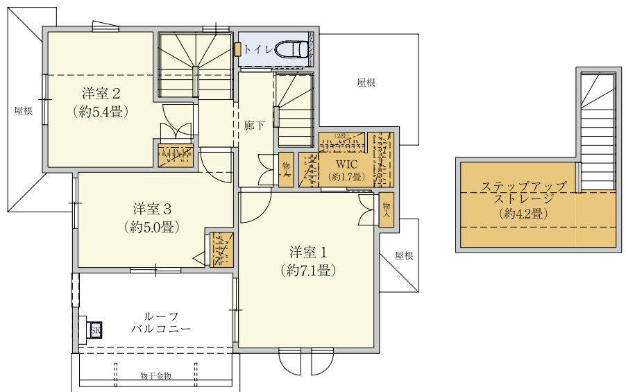
【2階平面図】
