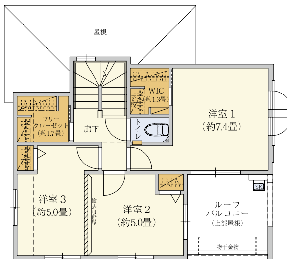
【2階平面図】
