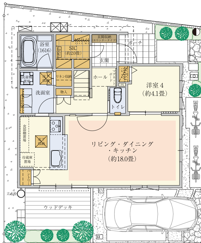
【1階平面図】
