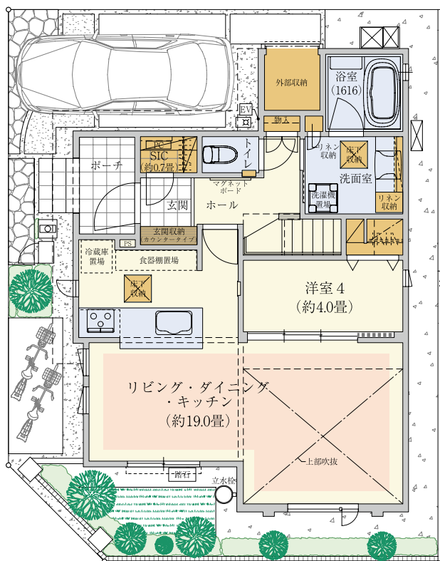
【1階平面図】
