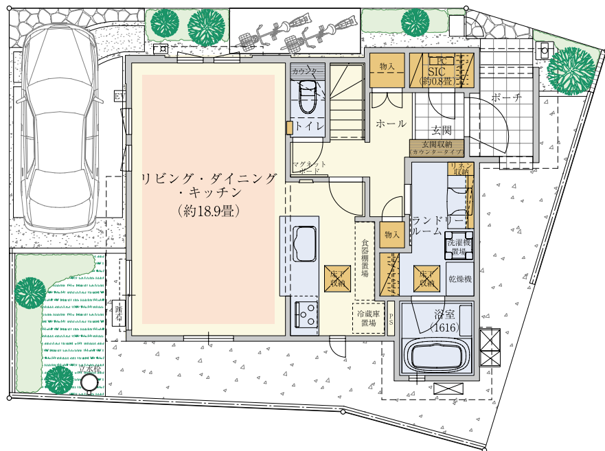
【1階平面図】
