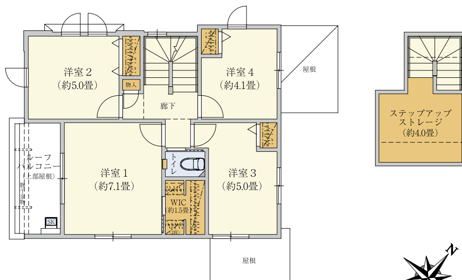
【2階平面図】
